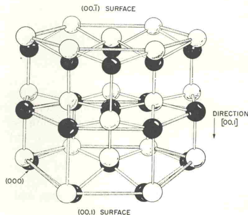
Fig. 1. Wurtzite structure
